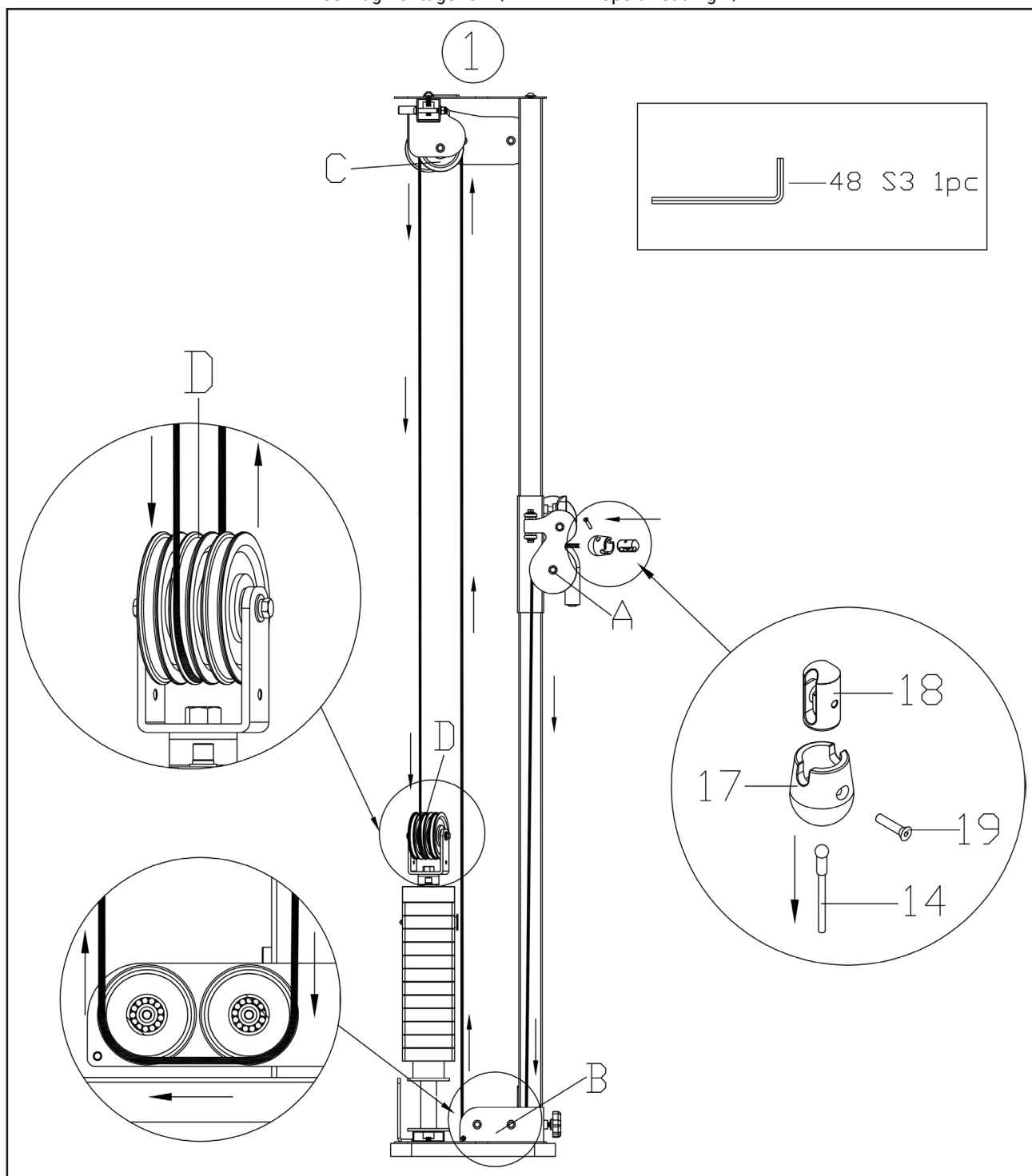
Seilzugmontage für 1/2
