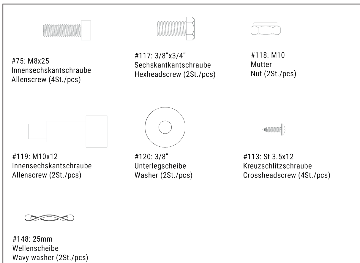
Benötigte Teile für Schritt 3 Needed parts for Step 3
