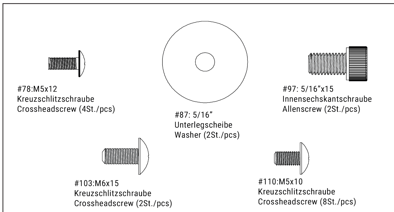
Benötigte Teile für Schritt 2 Needed parts for Step 2
