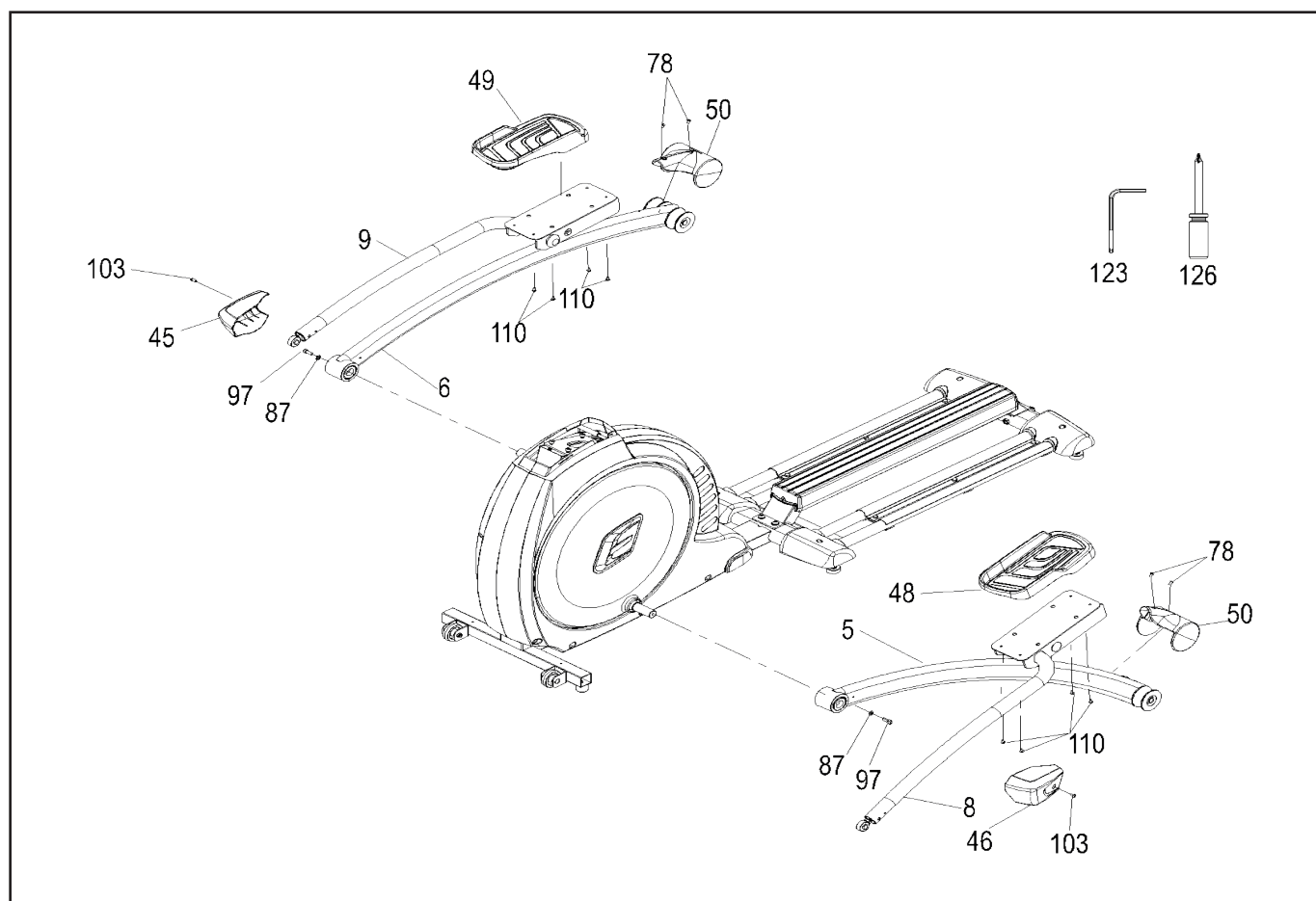
Benötigte Teile für Schritt 2 Needed parts for Step 2
